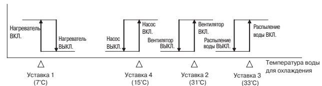
Регулирование T3
